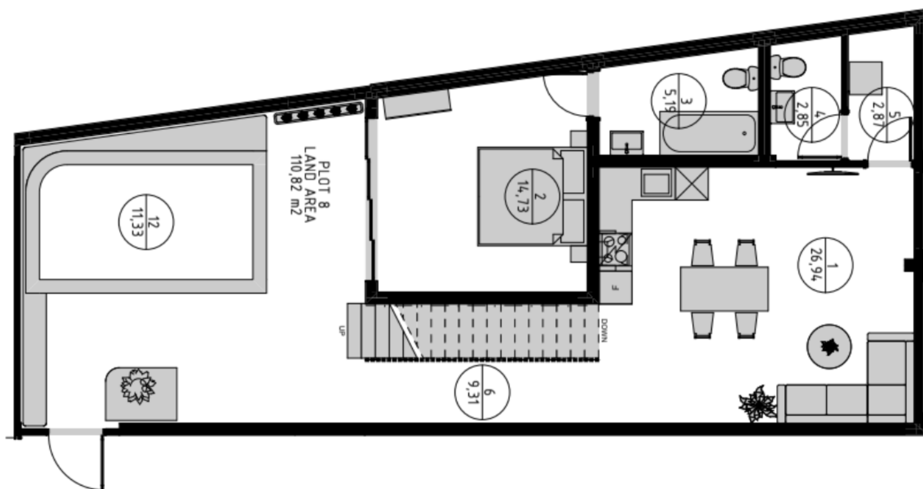
0 Этаж
