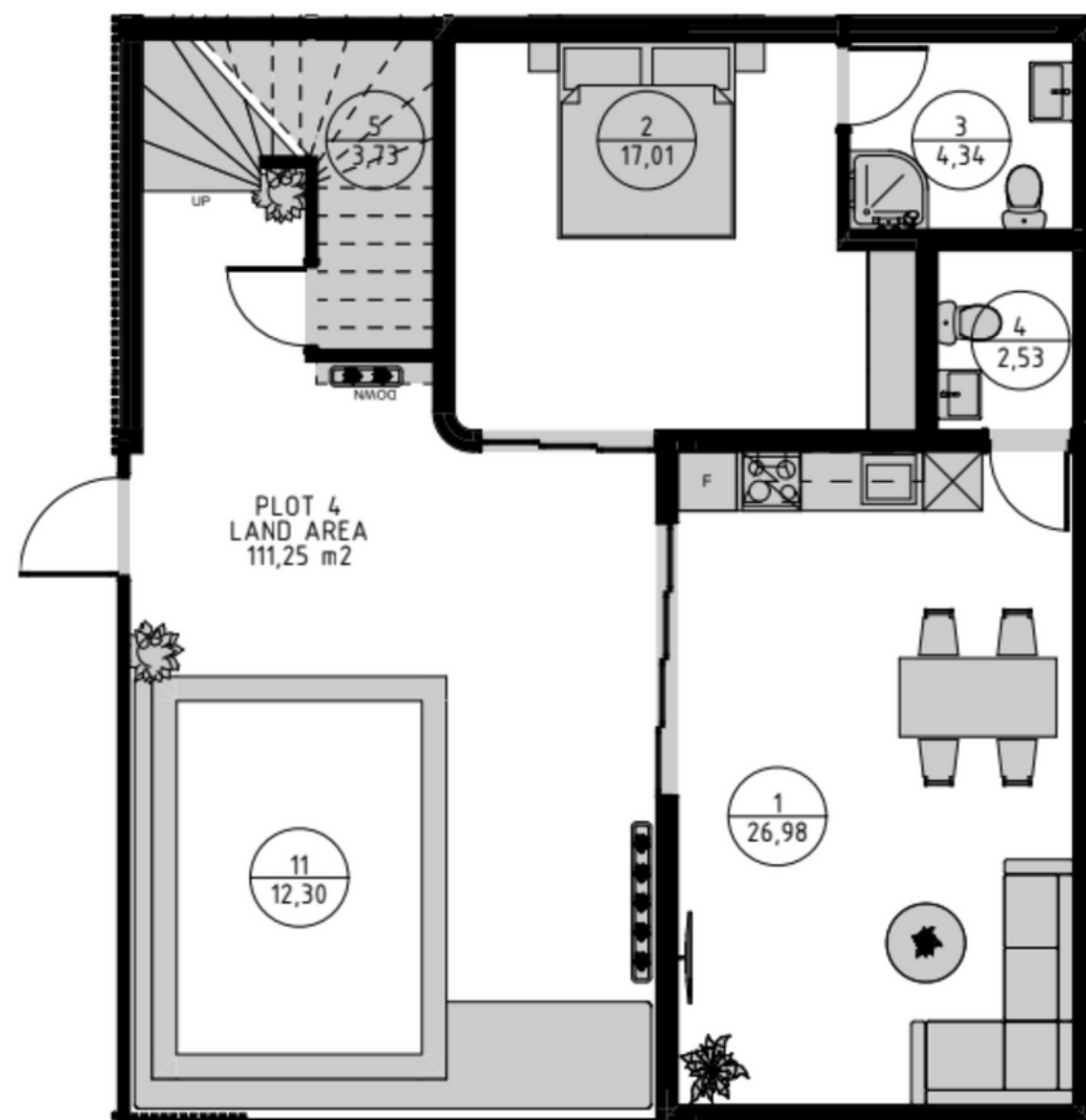
0 Этаж
