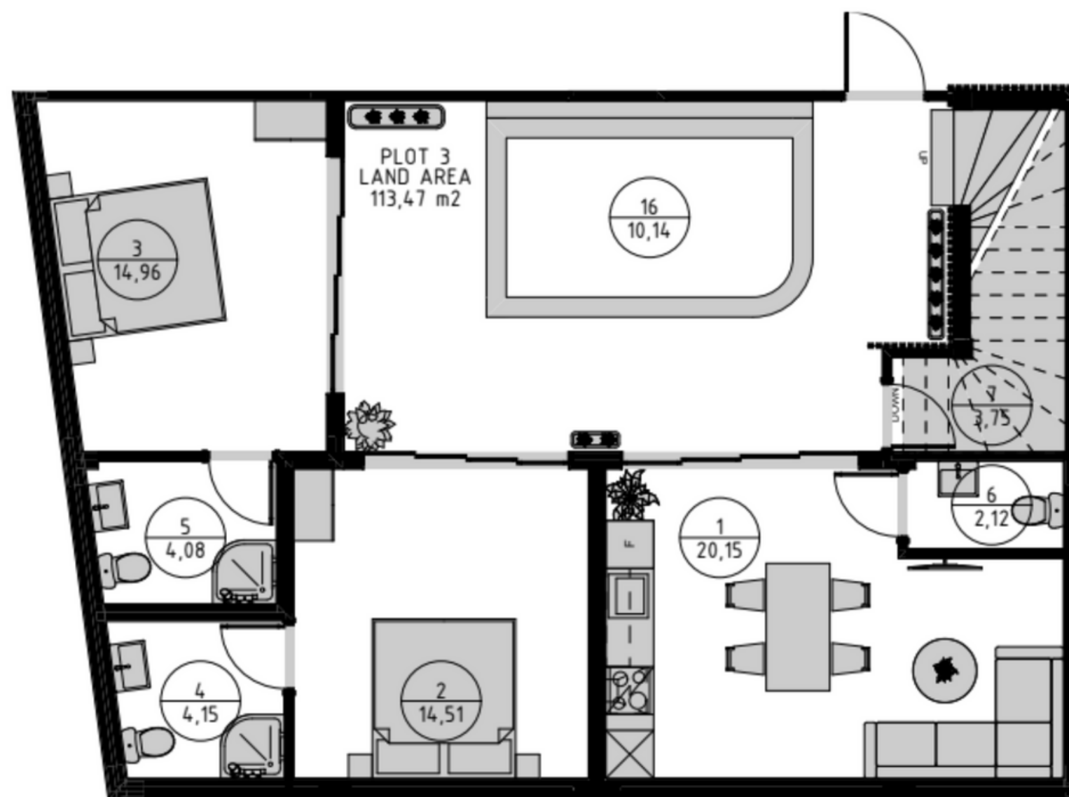
0 Этаж
