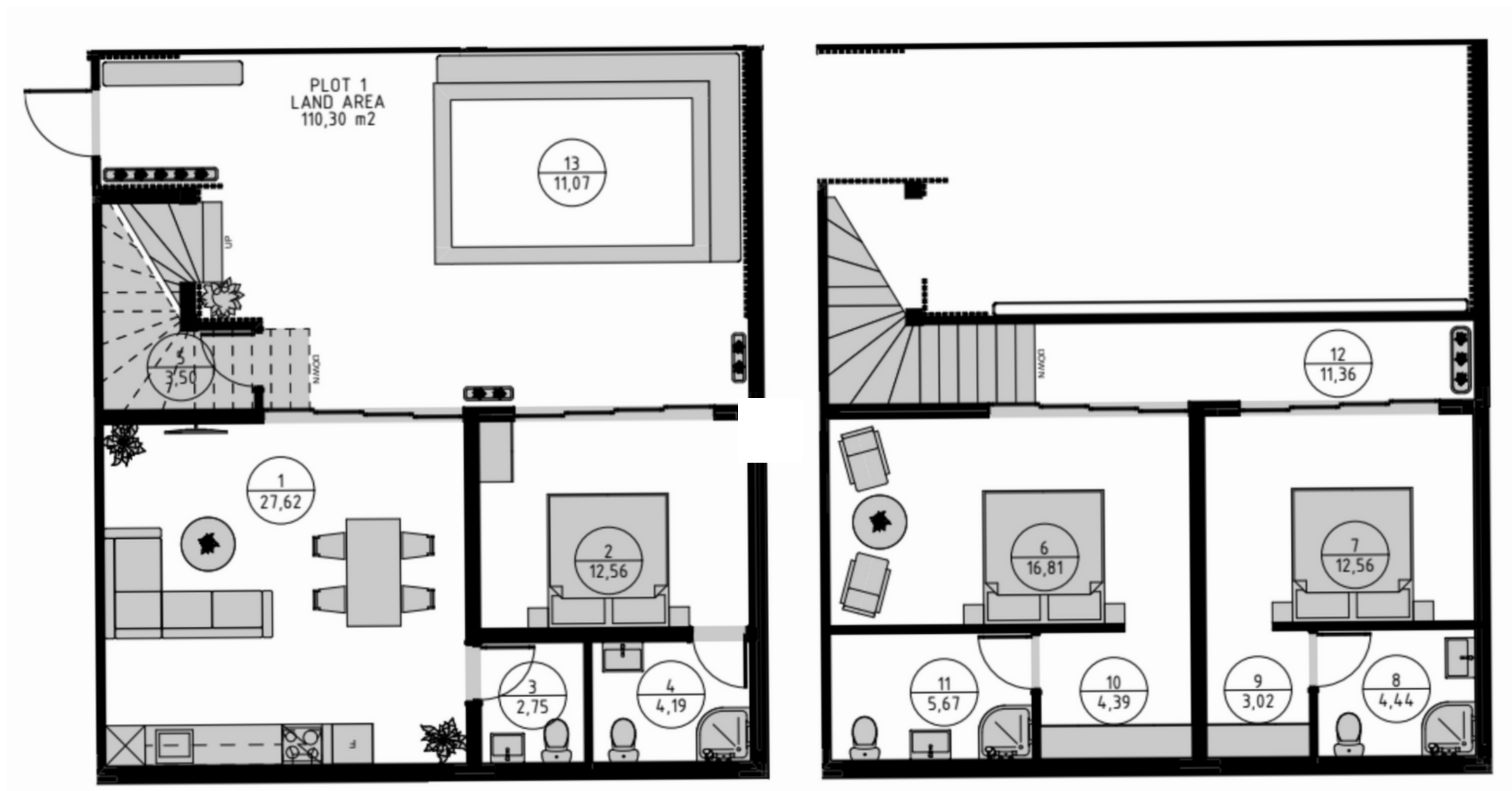
0 Этаж
